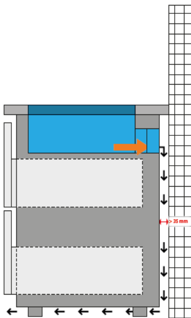
Umluftbetrieb ungeführt ab 60 cm Arbeitsplattentiefe möglich Abstand zur Wand, mind. 35 mm
