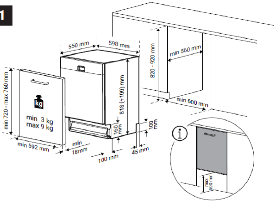
Nischentiefe 560 mm (exklusive Möbelfront)
